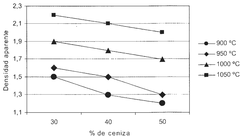
Figura N° 13: Variación de la densidad aparente vs. % de ceniza
