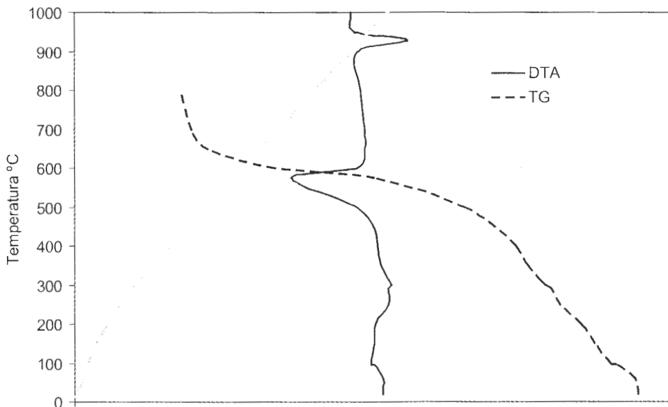
Figura N° 10: Análisis térmico de la laterita (DTA y TG)
