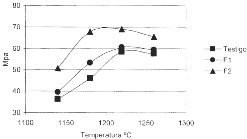
Figura N° 26 : Resistencia a la flexión (según norma IRAM 11827) vs. temperatura (valores promedio sobre 10 determinaciones) :
