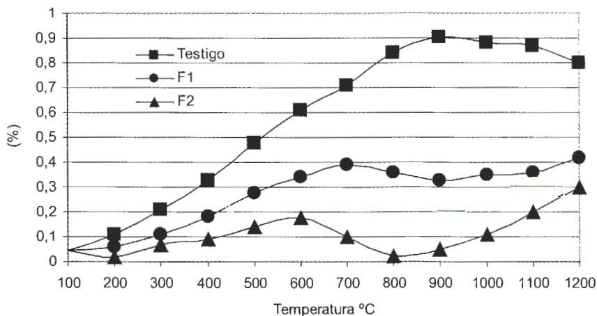
Figura N° 23: Porcentaje de dilatación vs. temperatura.
