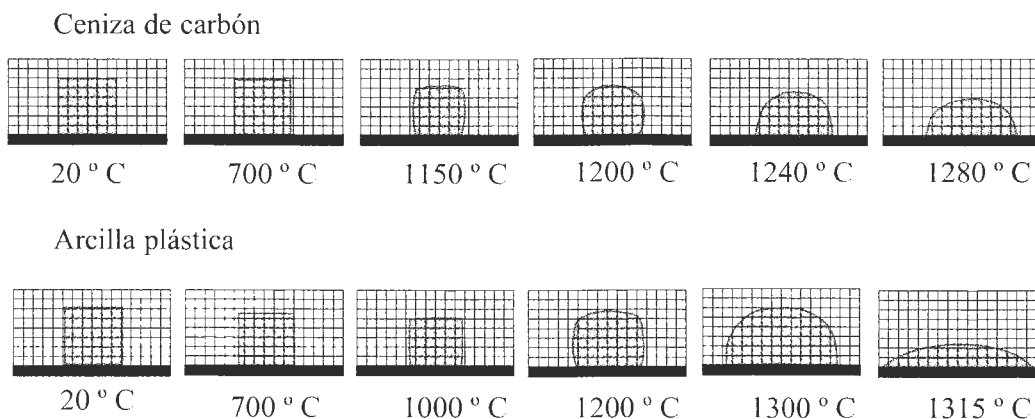
Figura N° 21: Microscopía de calentamiento
