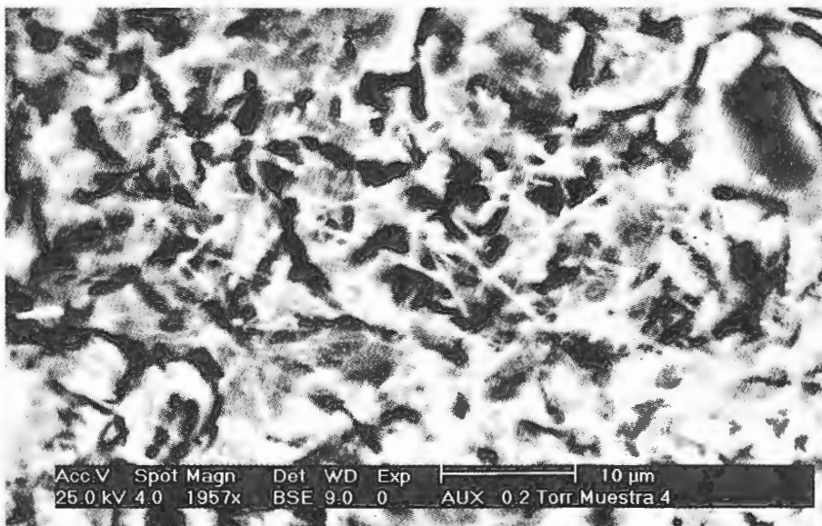
Figura N°20 : Microestructura de la muestra N°4
