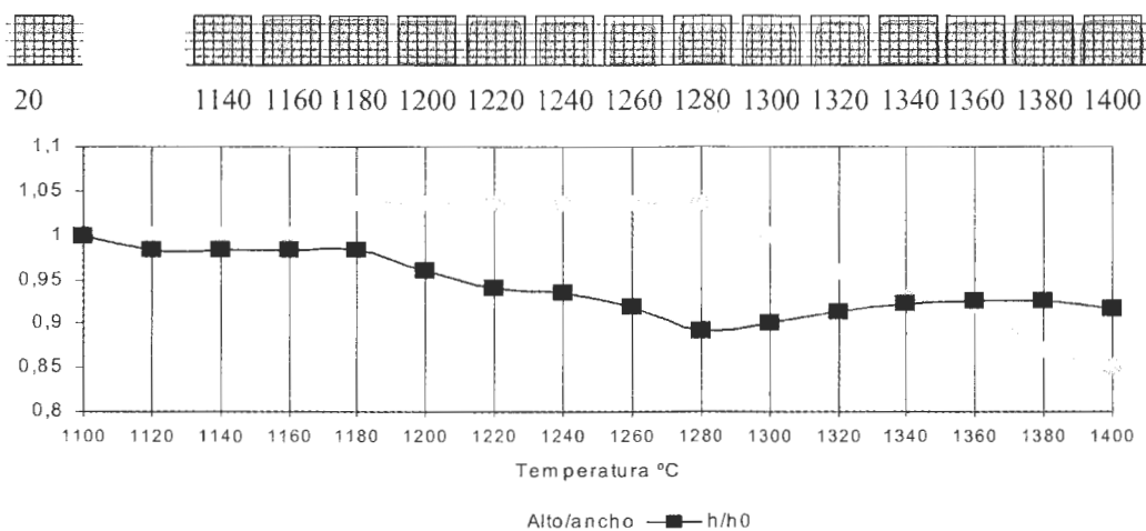
Figura N° 9: Microscopía de alta temperatura
