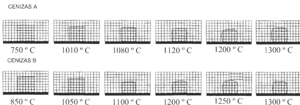
Figura N° 12 : Microscopía de calentamiento de las cenizas
