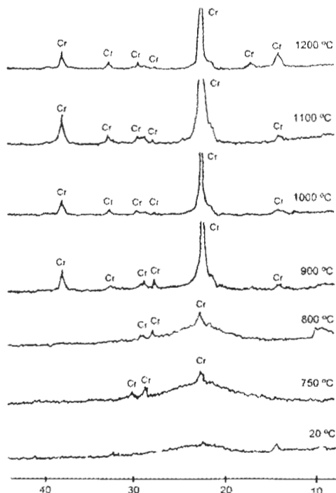
Figura N° 8: Diagramas de difracción de rayos X de las muestras calcinadas
