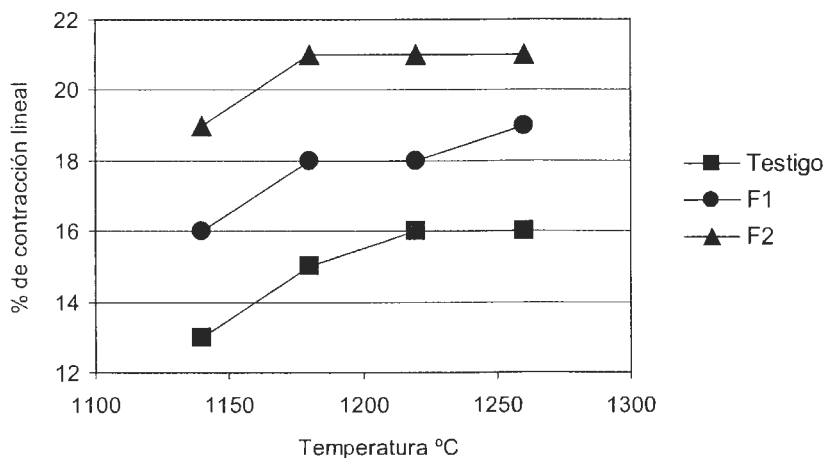
Figura N° 25 : Contracción lineal total vs. temperatura
