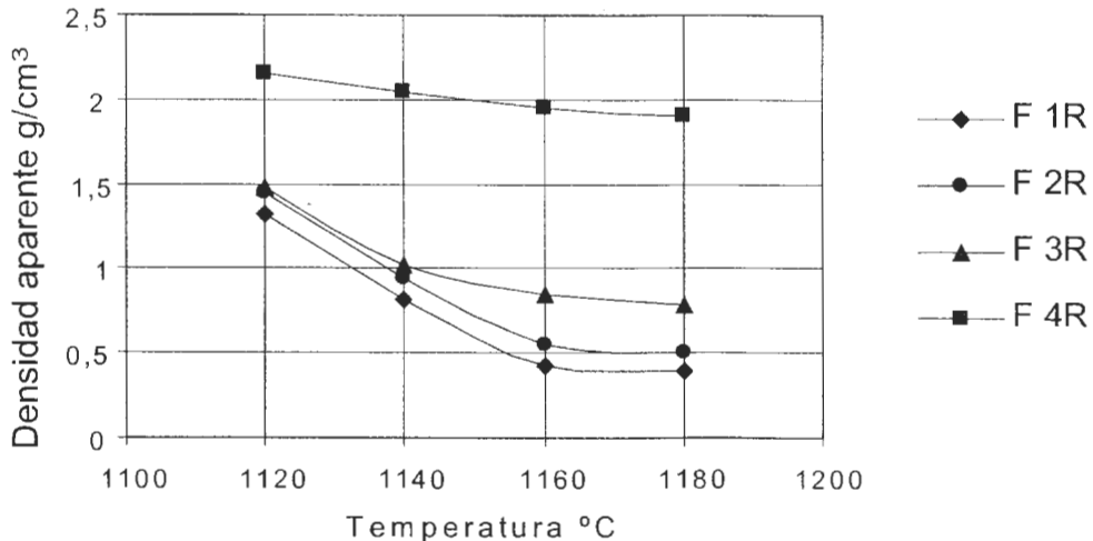
Figura N° 30: Variación de la densidad aparente de las muestras
