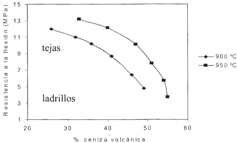
Figura N° 14: Variación de la resistencia a la flexión vs. % de ceniza
