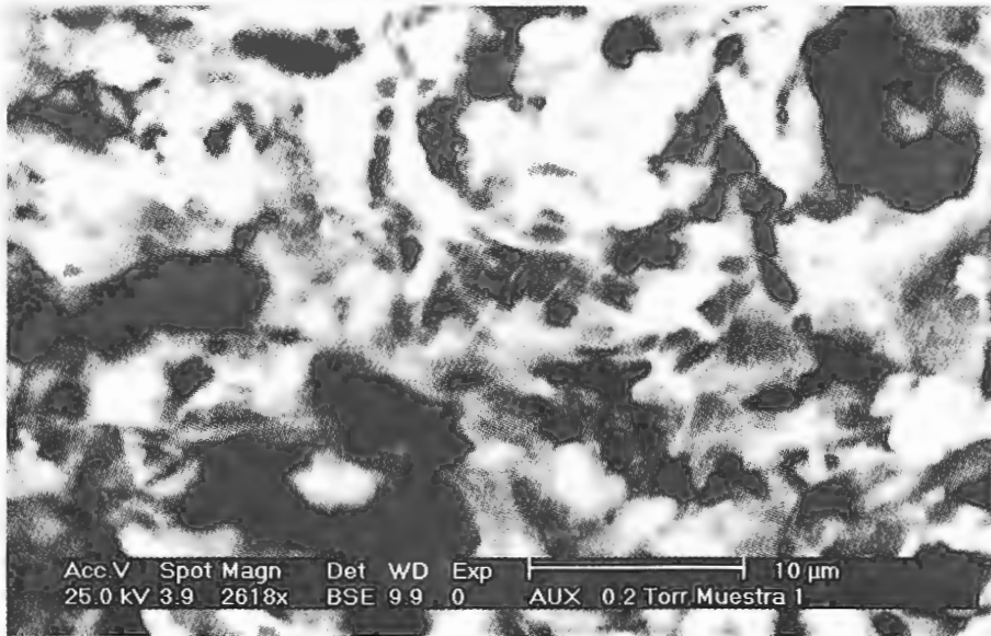
Figura N°19 : Microestructura de la muestra N°1
