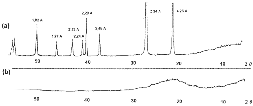
Figura N° 22: Difractograma de cuarzo (a) y ceniza (b)
