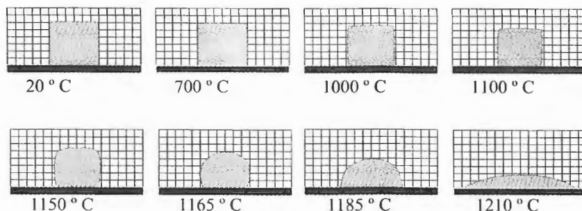
Figura N° 1: Microscopía de calentamiento
