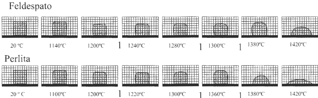
Figura N° 15: Microscopía de calentamiento
