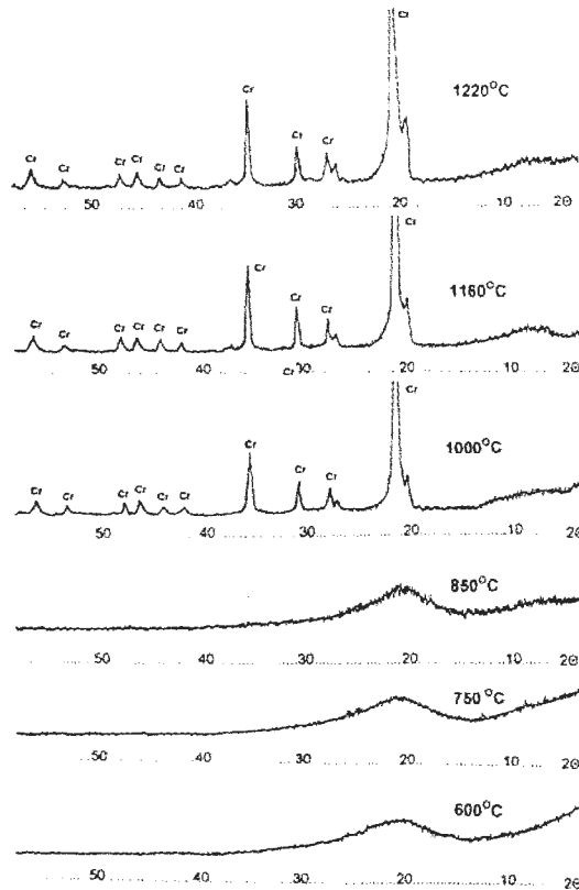
Figura N° 28: Difractogramas de la ceniza calcinada a diferentes temperaturas
