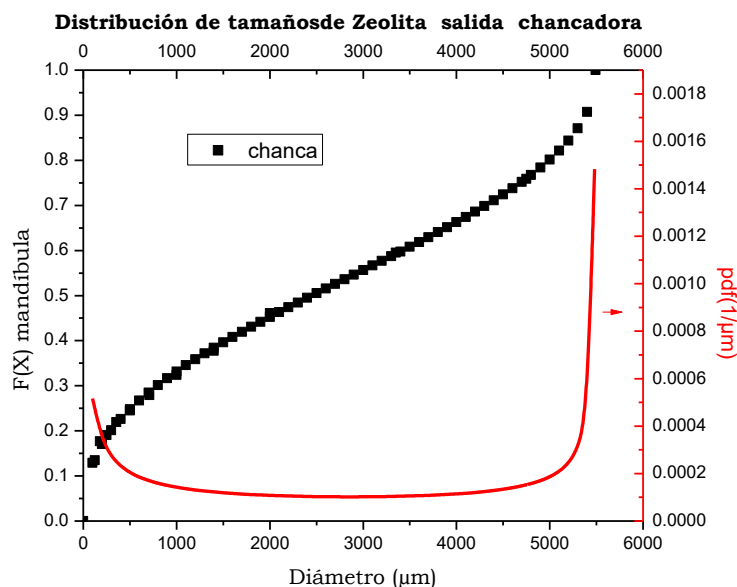
Figura 3: Distribución de tamaños de Zeolita en la salida de la chancadora - trituradora
